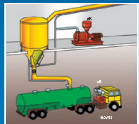
Fluidizing
